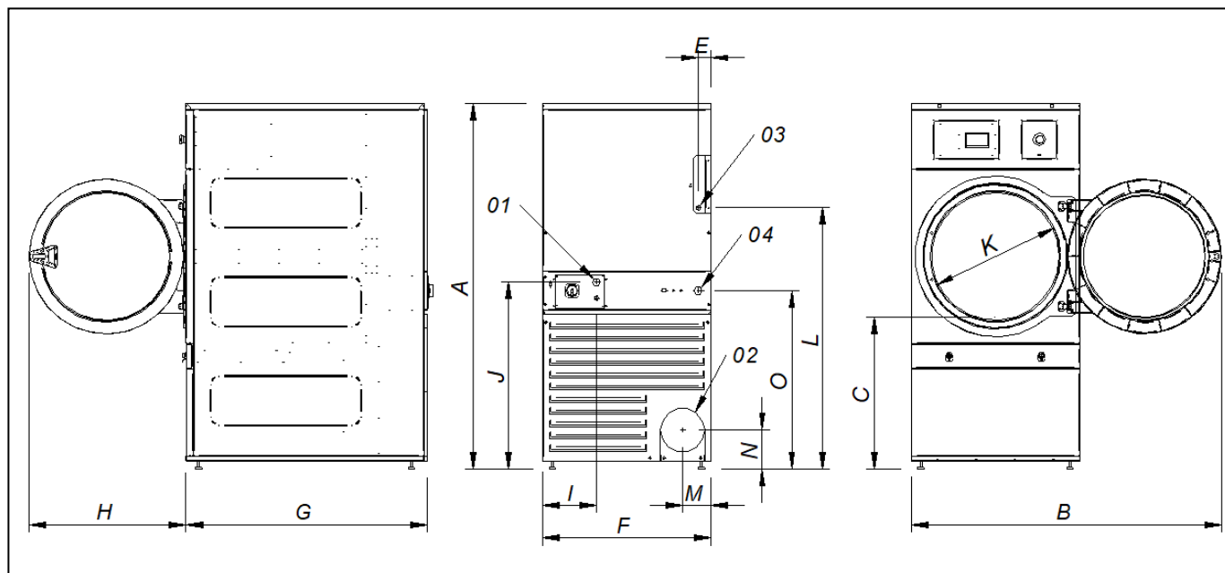
DIMENSIONS GÉNÉRALES
