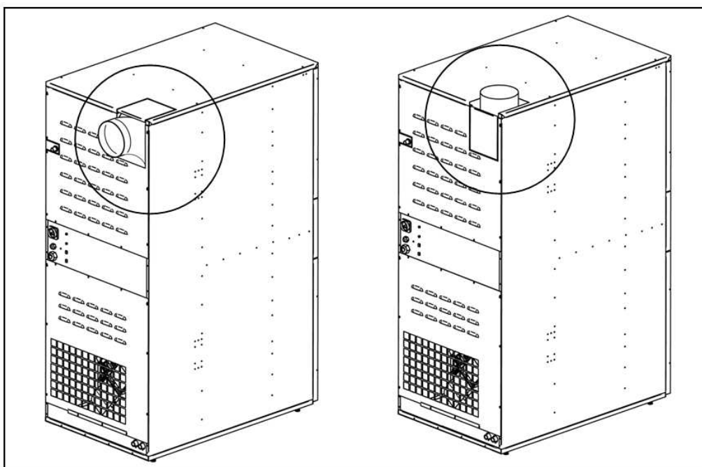
Option of the 90° (1.57 rad) L-bend
