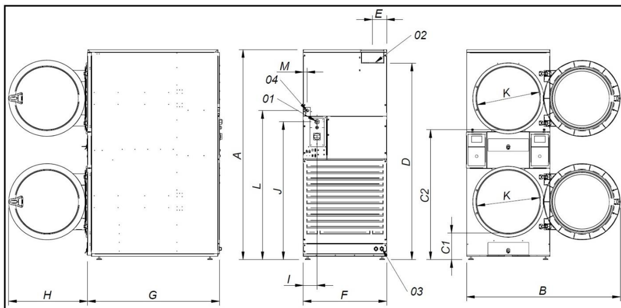
DIMENSIONS GÉNÉRALES (indiquées en mm) :
