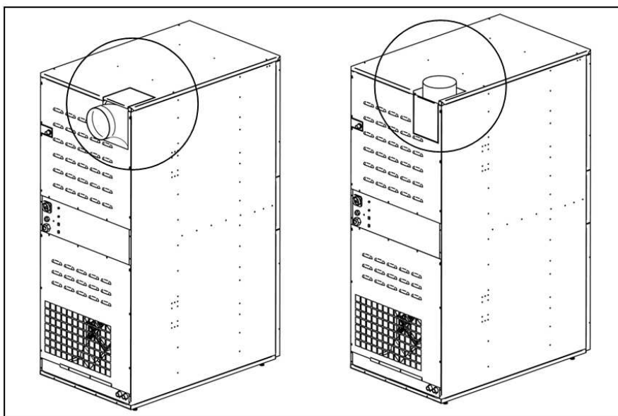
Option of the 90° (1.57 rad) L-bend
